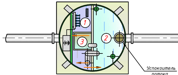
Разрез А-А (1:10)
