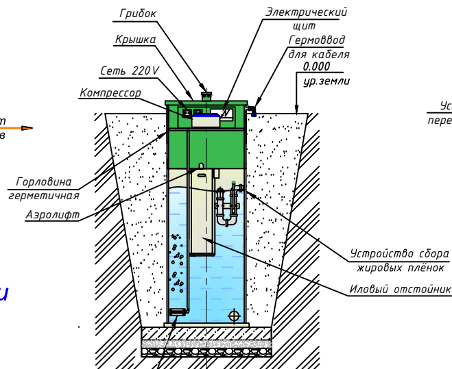
Разрез В-В
